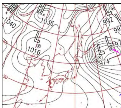
収束線形成
