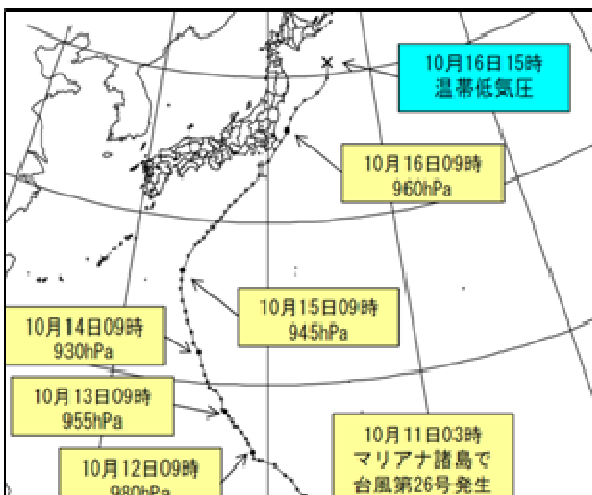
台風経路図（気象庁ホームページ）
