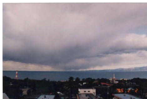
北東風
